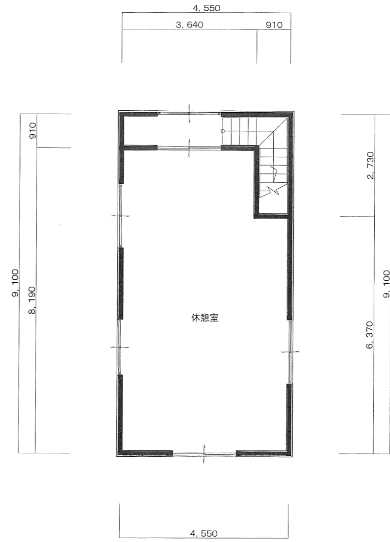
2階平面図
