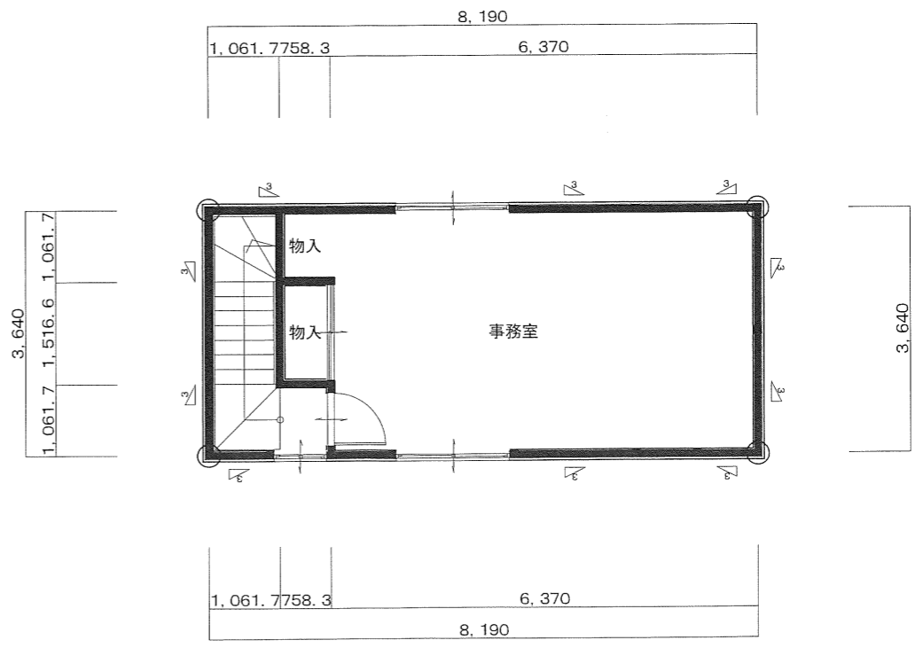
2階平面図
